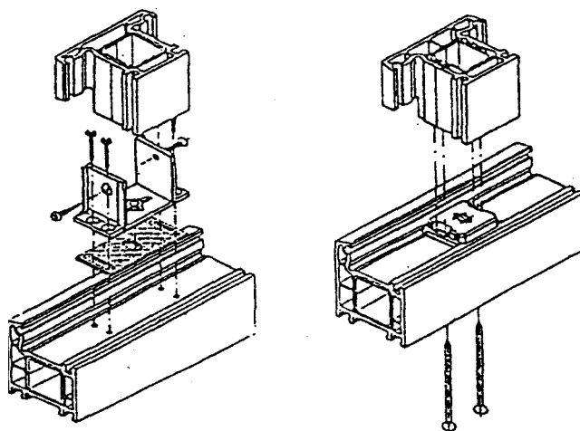
Рисунок 8 — Примеры крепления импостов
