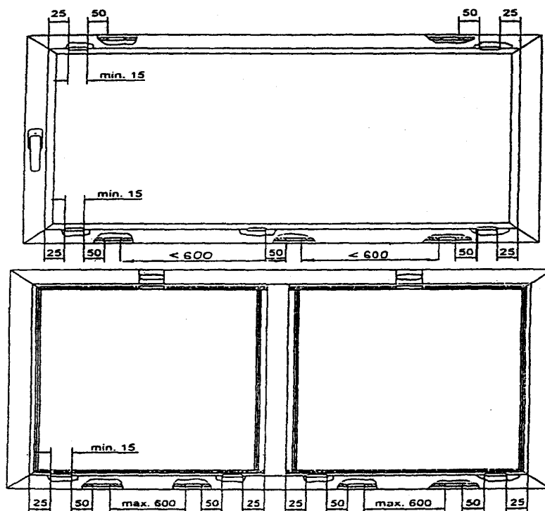
Рисунок В.2 — Расположение функциональных отверстий
