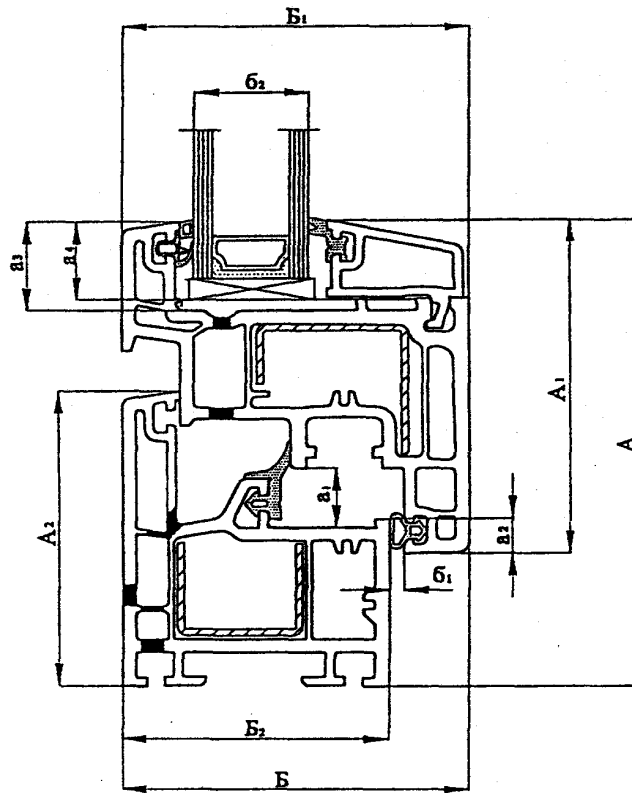
A — высота комбинации профилей; A 1 — высота профиля коробки; A 2 — высота профиля створки; B — ширина комбинации профиля; B 1 — ширина профиля створки;
