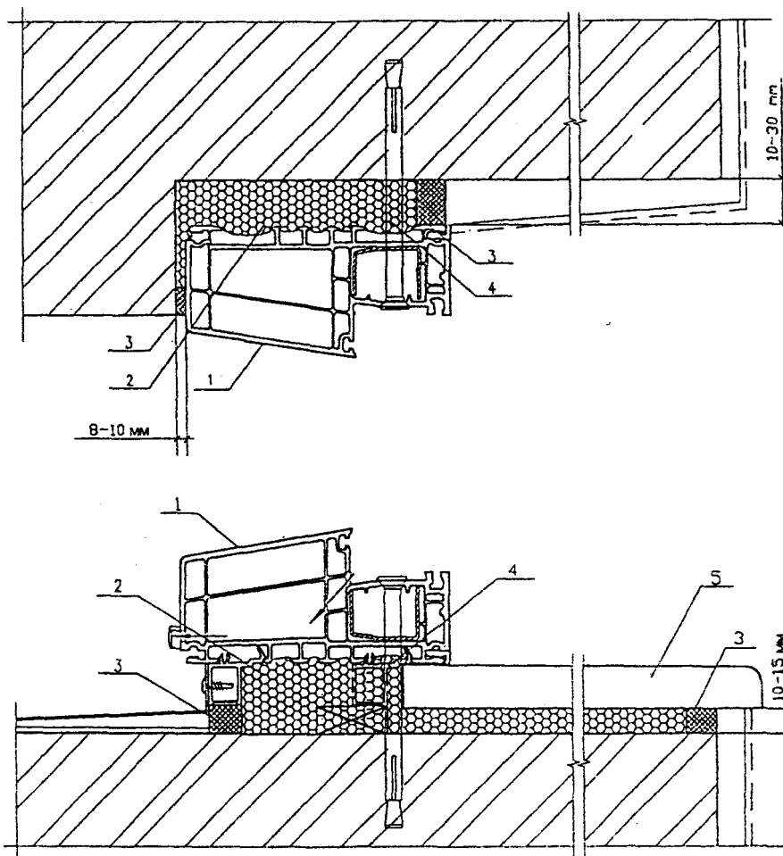
Рисунок Г.1 — Пример монтажного узла оконного блока
