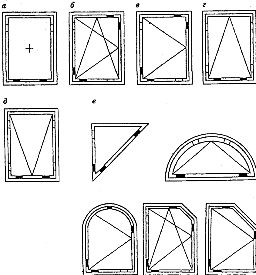
Виды оперывания оконных блоков: а — неоткрывающиеся; б — поворотно-откидное; в — поворотное (распашное); г — откидное; д — подвесное; е — установка подкладок в фигурных оконных блоках
