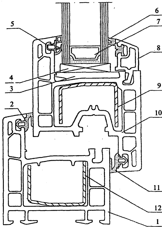
1 — коробка; 2 — прокладка наружного уплотнения; 3 — базовая подкладка; 4 — опорная подкладка; 5 — наружная уплотняющая прокладка стеклопакета; 6 — внутренняя уплотняющая прокладка стеклопакета; 7 — стеклопакет; 8 — штапик; 9 — усиленный вкладыш створки; 10 — створка; 11 — прокладка внутреннего уплотнения; 12 — усиленный вкладыш коробки
