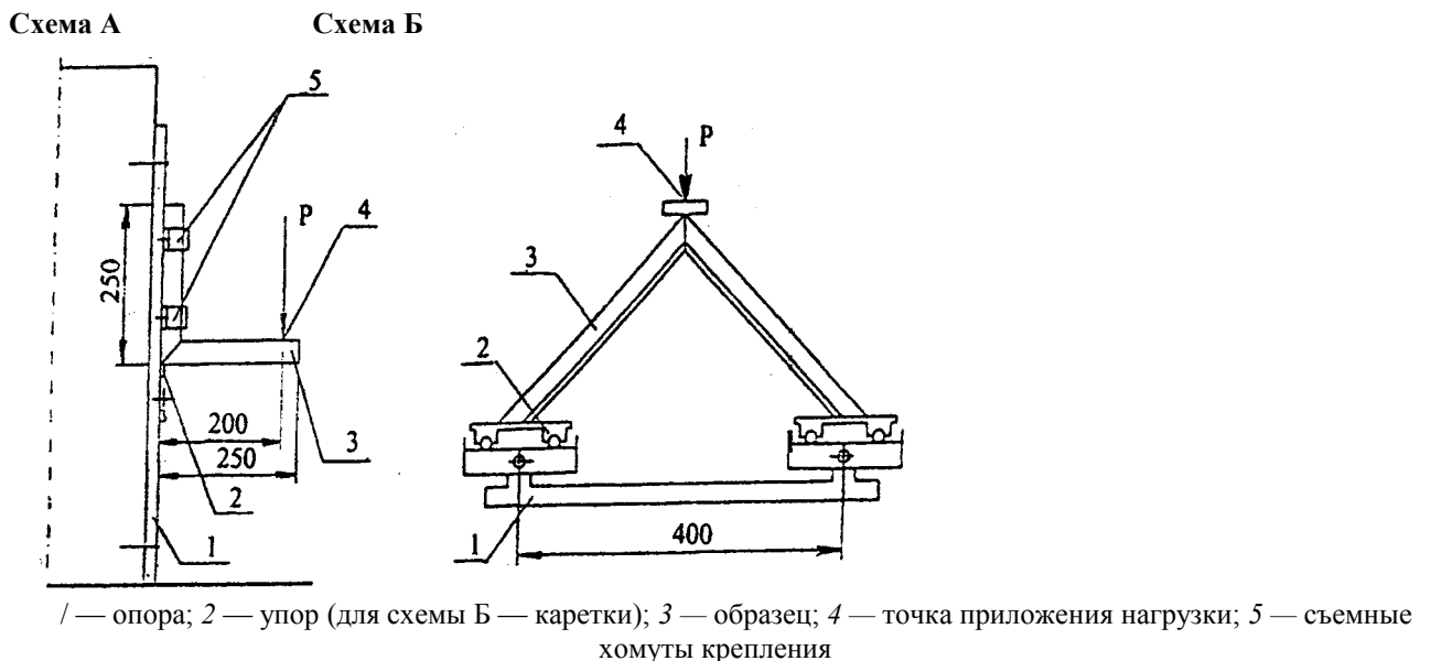
Рисунок 9 — Схемы приложения нагрузок при определении прочности угловых сварных соединений
