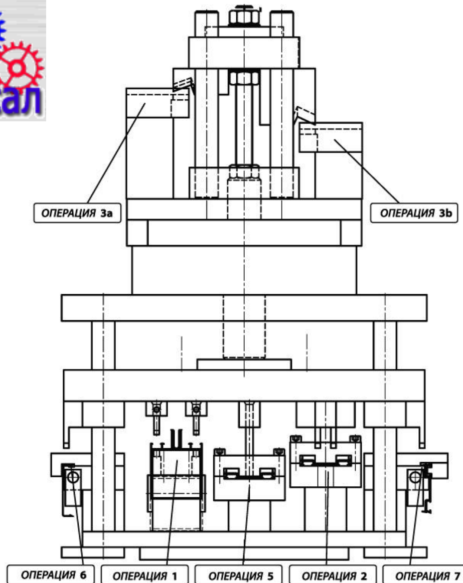
Матрица с пневматическим прессом KRF
