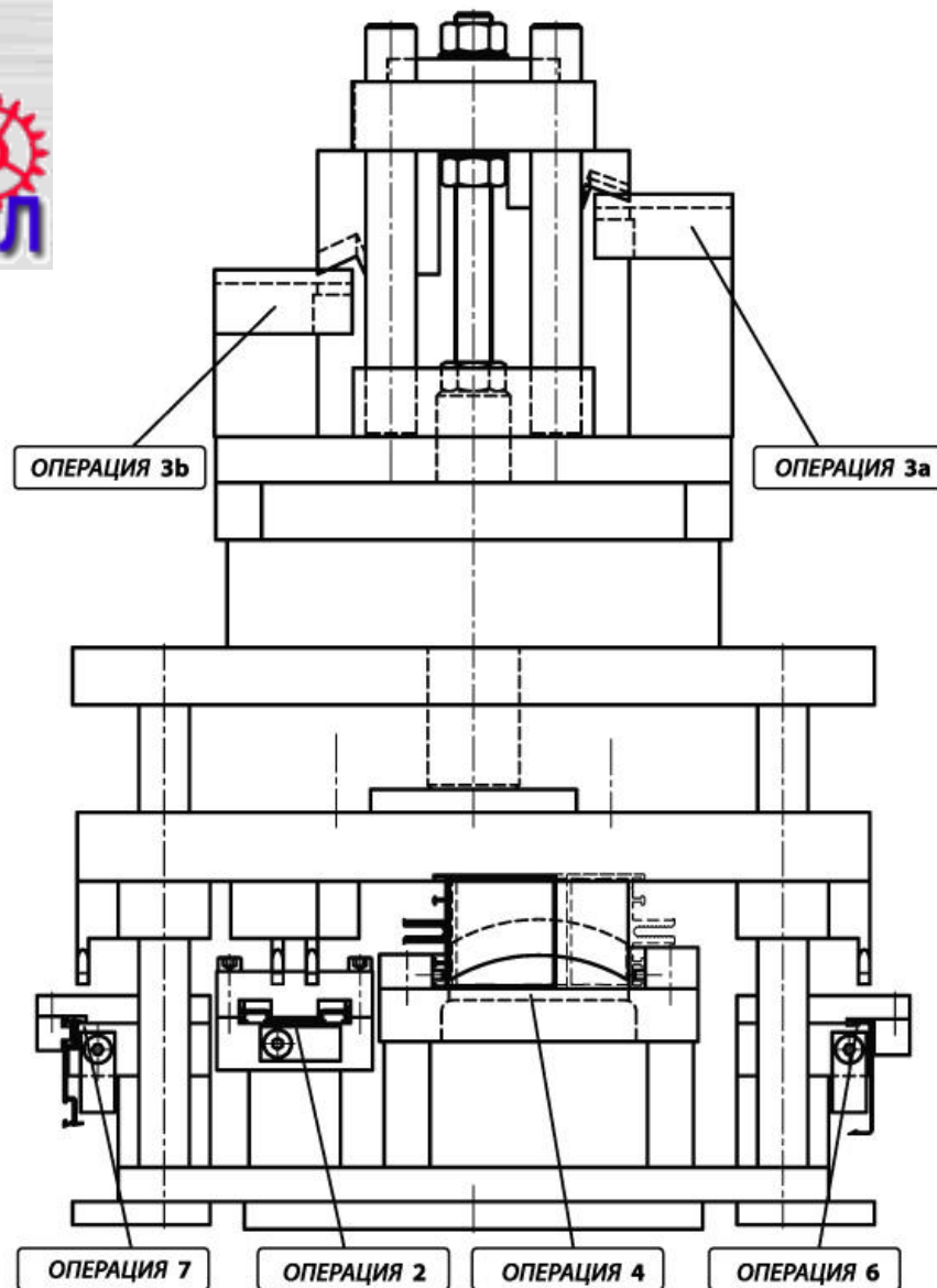
Матрица с пневматическим прессом KRF
